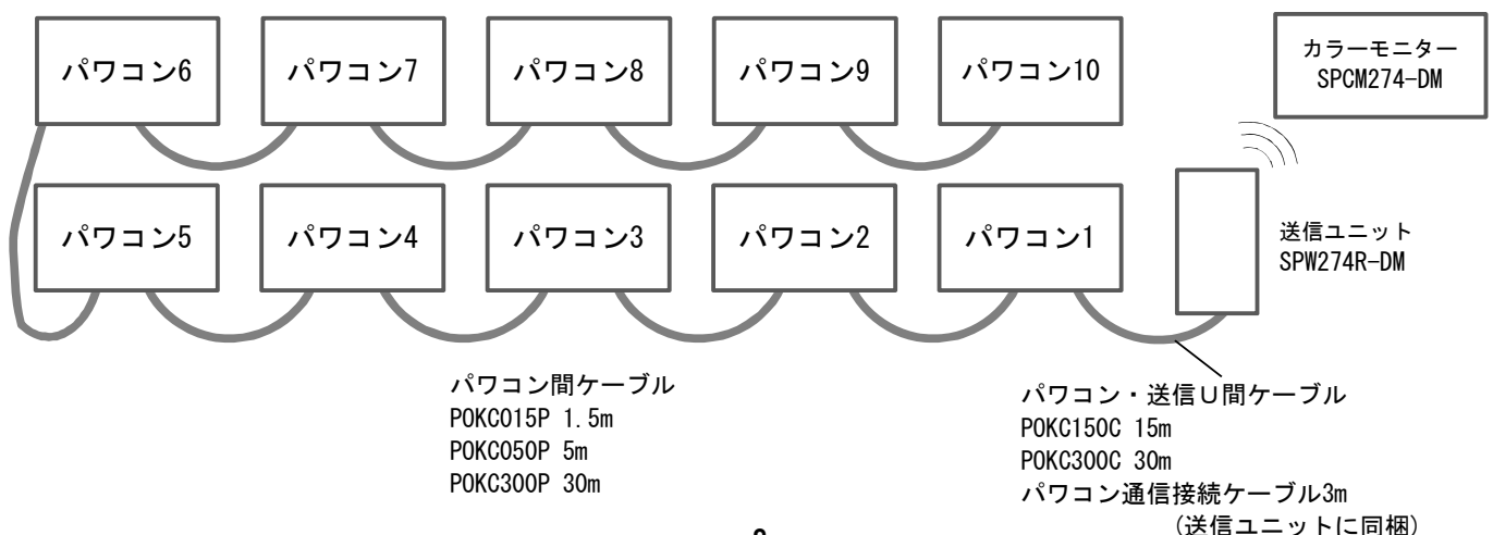
通信ケーブル配線図
