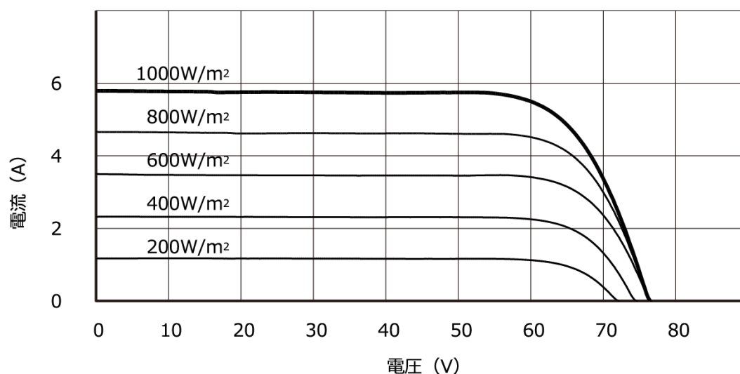
放射照度毎の I-V 特性（@25℃）
