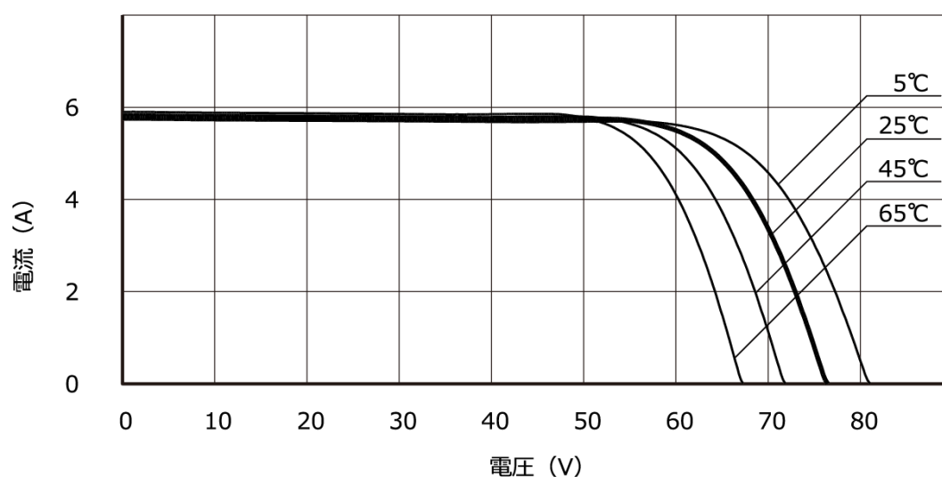
温度毎の I-V 特性（@1000W/m²）
