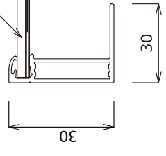
アルミフレーム断面
