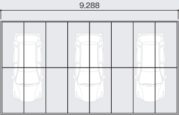
2段8列
