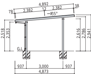
側面図 [1台用]
