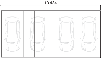
2段9列
